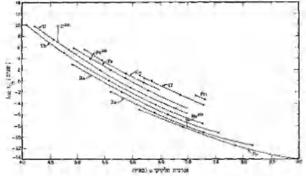
ציור 4. היחס בין זמן מחצית החיים לבין האנרגיה להתפרקות \alpha , t_{1/2} נמדד בשנים (פי Friedlander, ר' ביבל')
